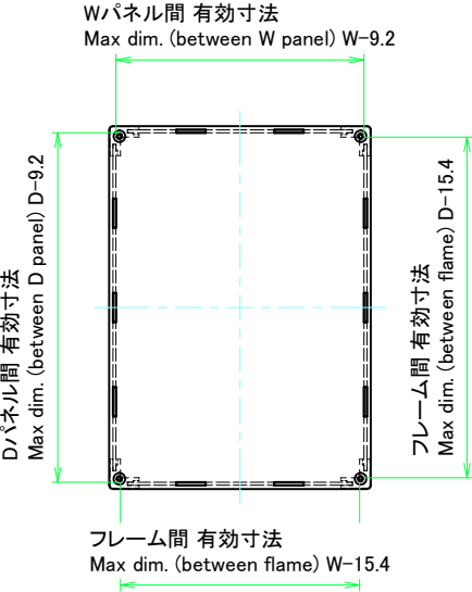
下カバー / Bottom cover
