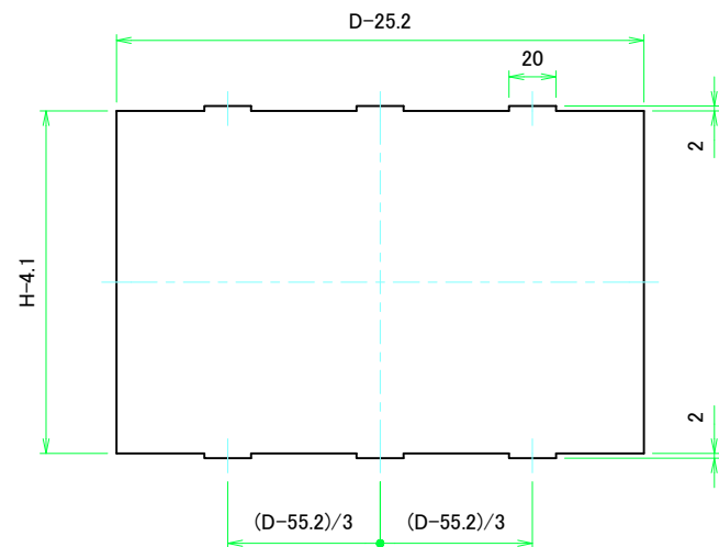
Dパネル1表面 / D Panel 1 Frontside
